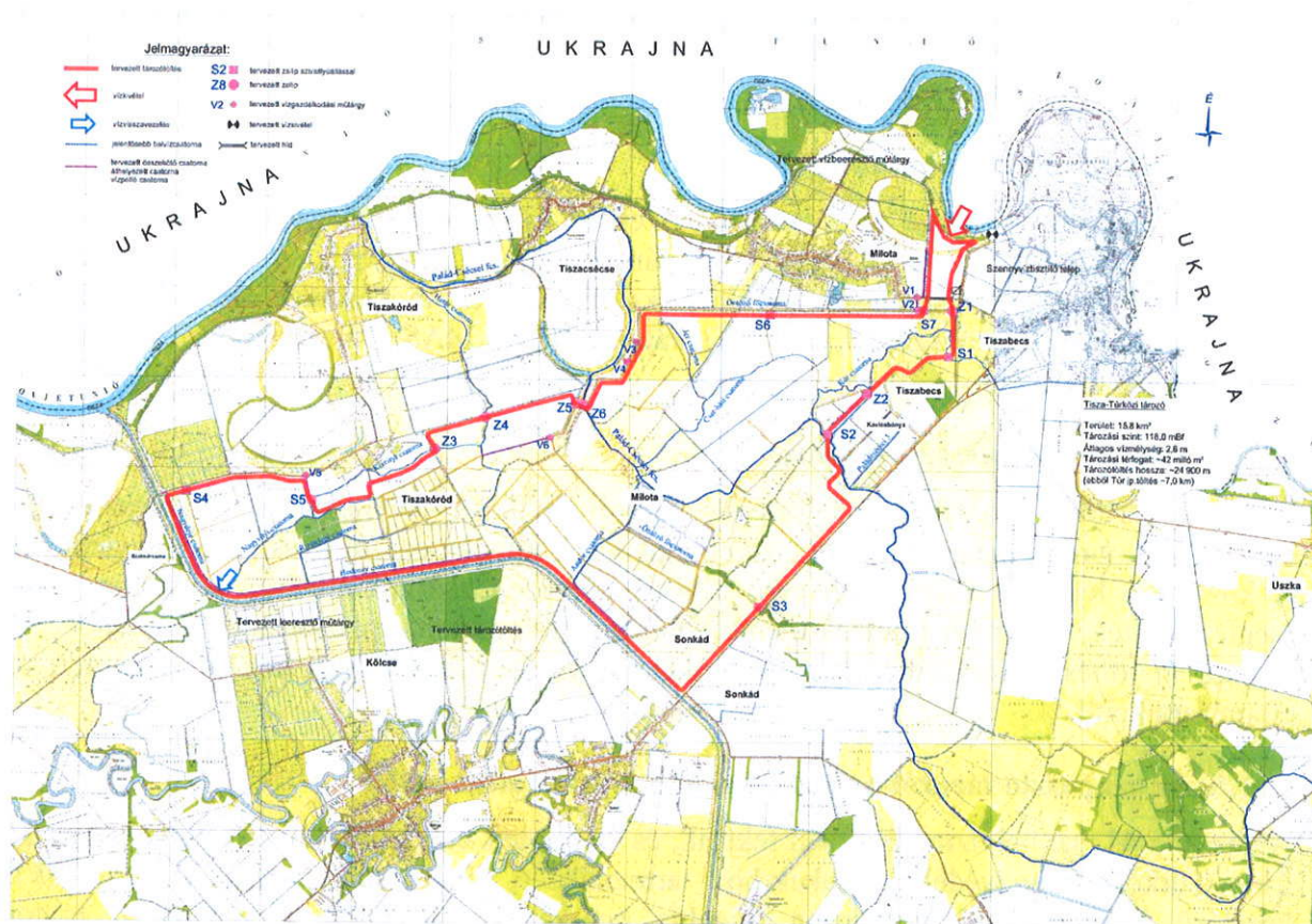
1. ábra Tisza-Túr árapasztó tározó területe
